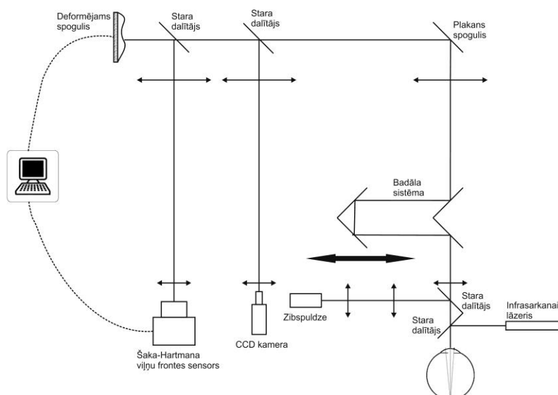
1. att. Optiskā shēma
